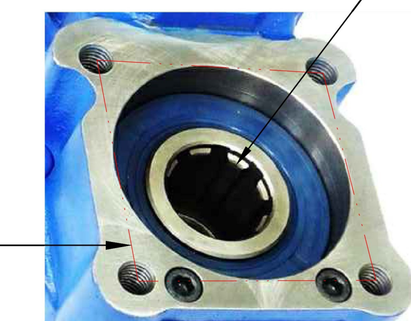
ISO 14 DIN 5462 8x32x36
